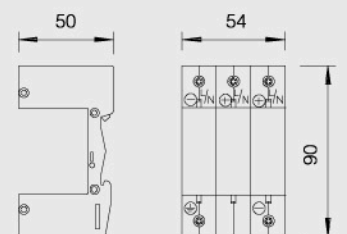
V20-C/3-PH尺寸图
