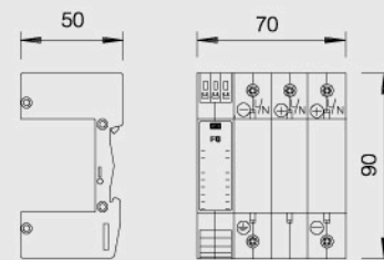
V20-C/3-PH-FS尺寸图
